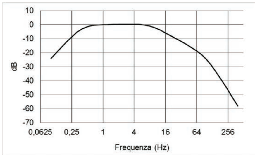
Curva di ponderazione W_c
