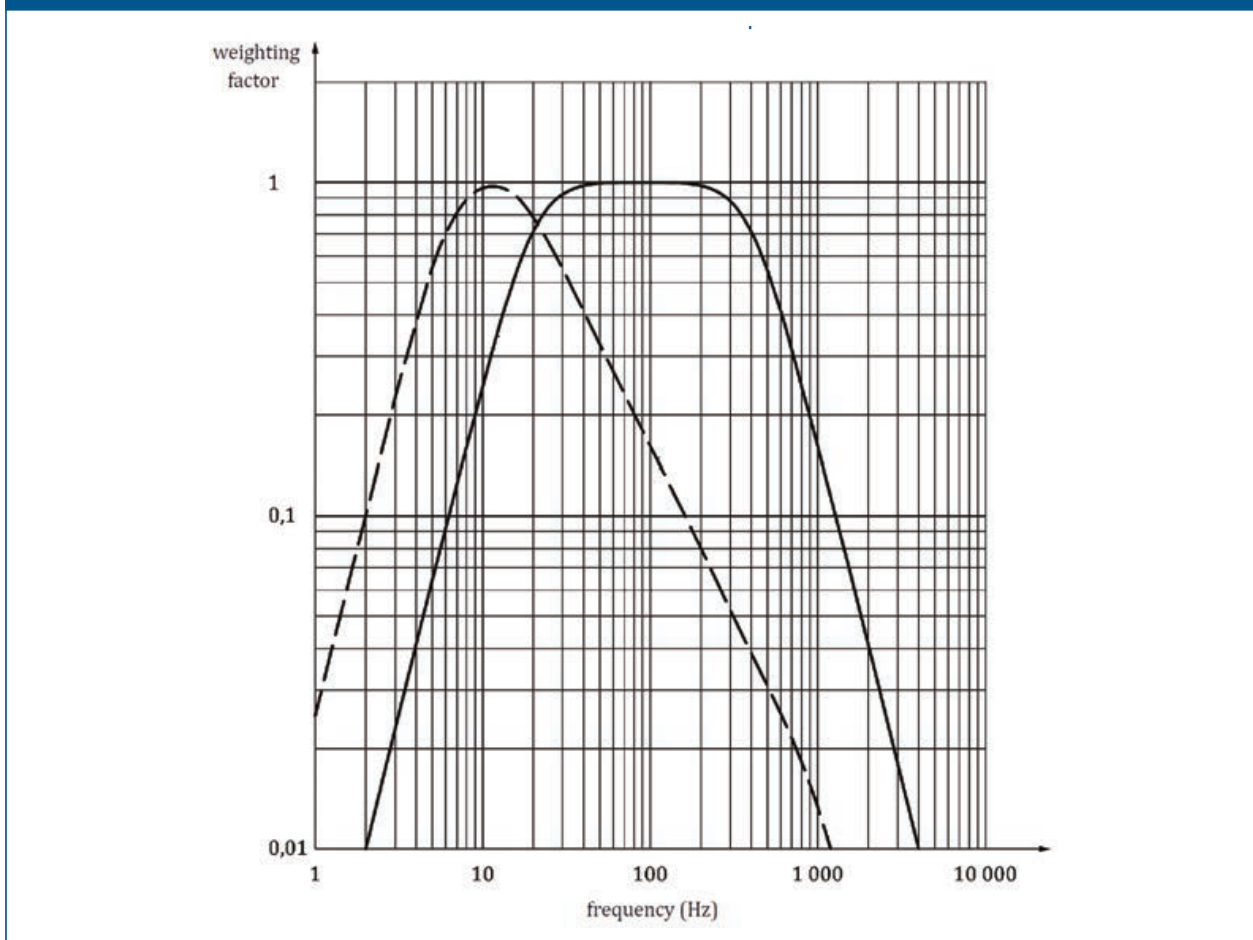
Figura 8 Andamento in frequenza delle curve di ponderazione W_p (linea continua) e W_h (linea tratteggiata).
